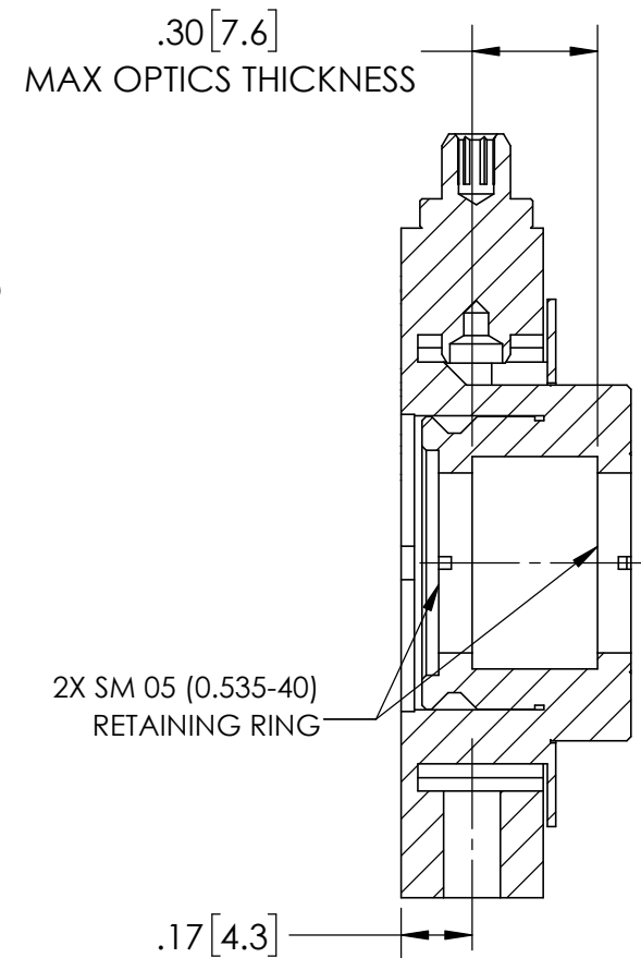
SECTION A-A
